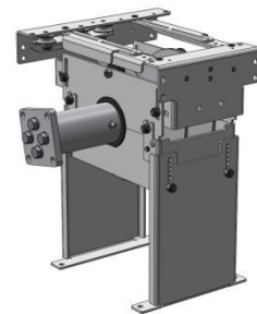
Mini Infinity 2 mechanism
