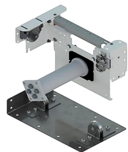
Vanishing Edge Assembly
